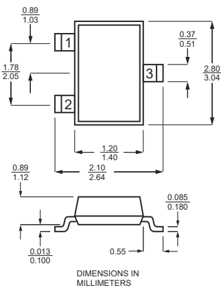
SOT-23
